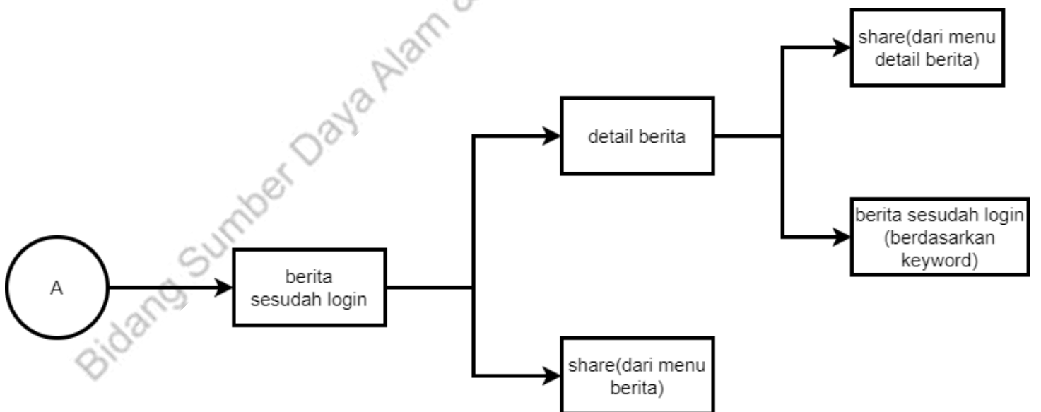
Gambar 20 UI Tree Berita (User)
