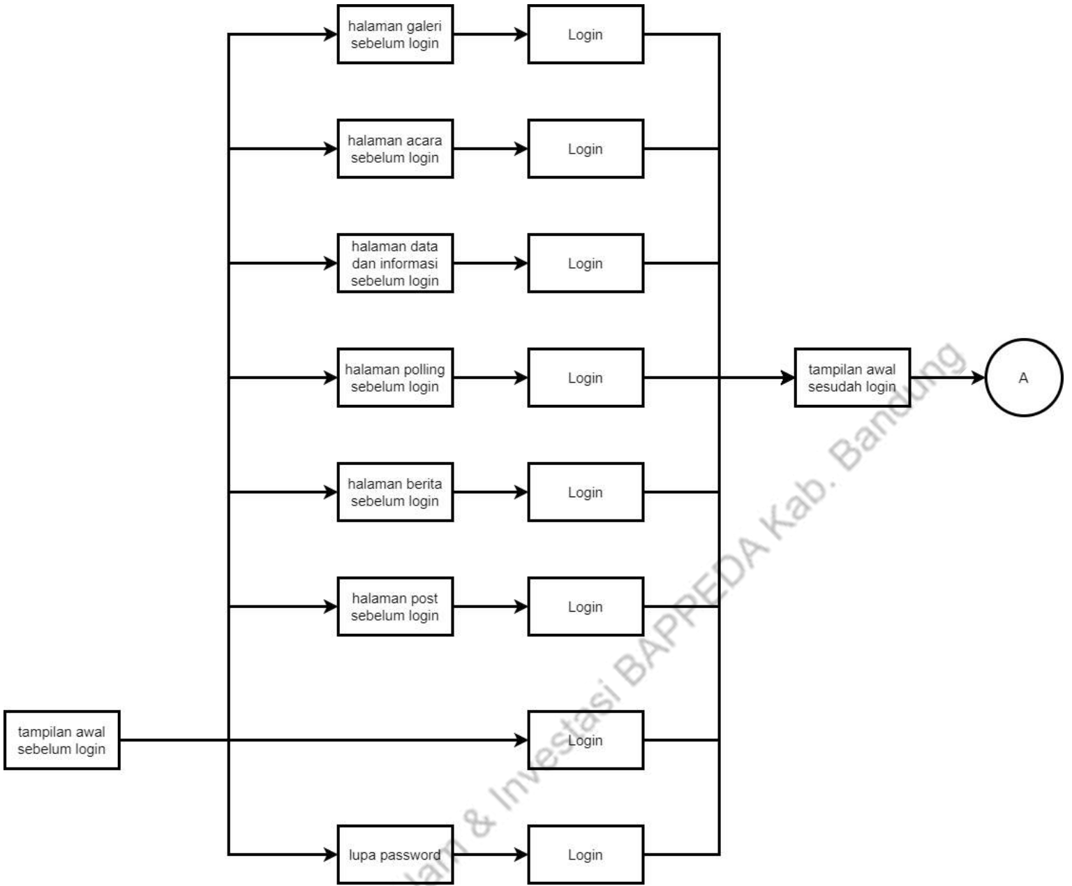
Gambar 7 UI Tree Sebelum Login (Admin)
