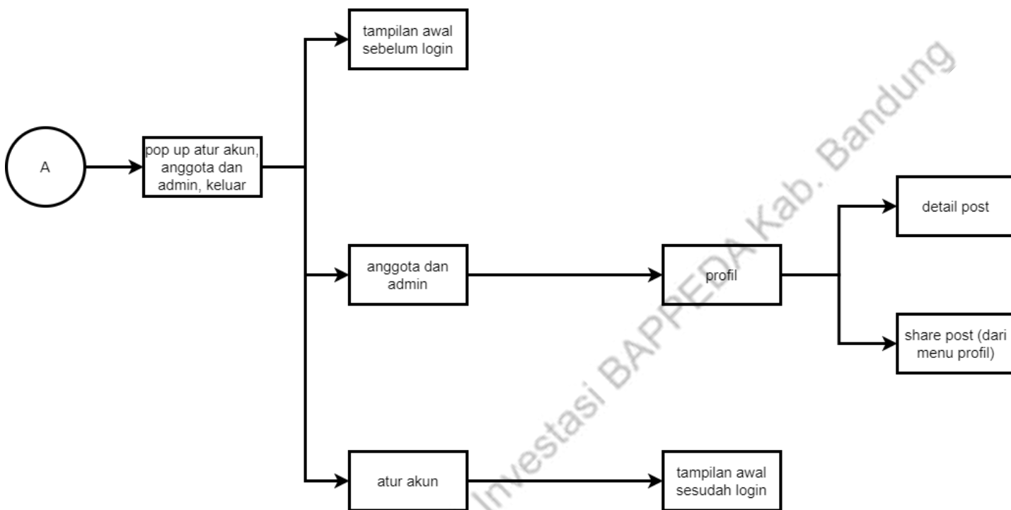
Gambar 27 UI Tree Akun (User)
