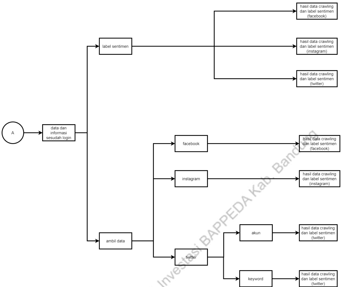
Gambar 12 UI Tree Data dan Informasi Bagian 2 (Admin)
