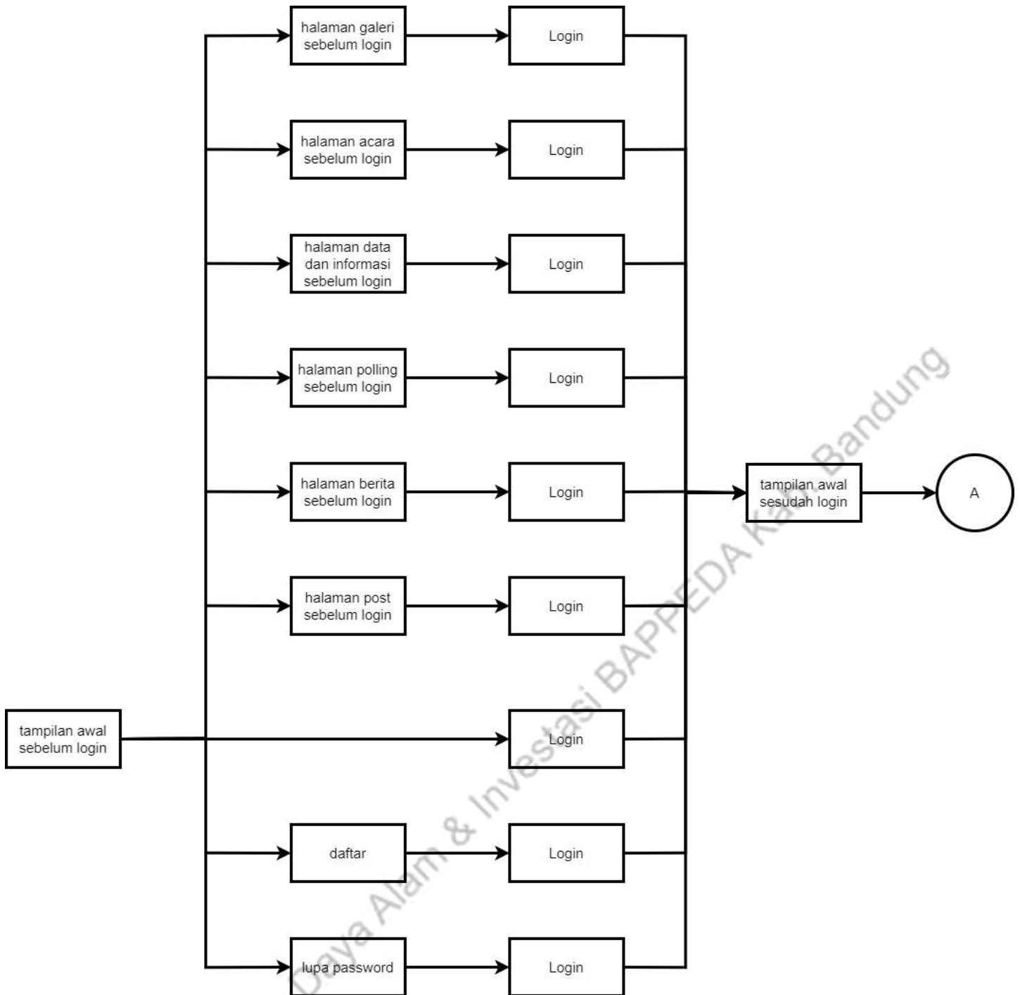
Gambar 18 UI Tree Sebelum Login (User)
