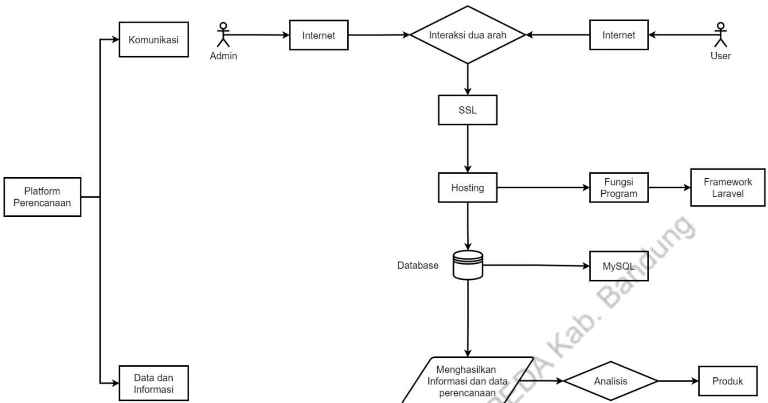
Gambar 6 Gambaran Umum Rencana Aplikasi
